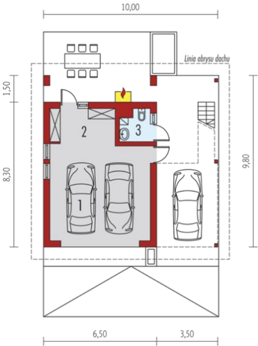
Rzut parteru
