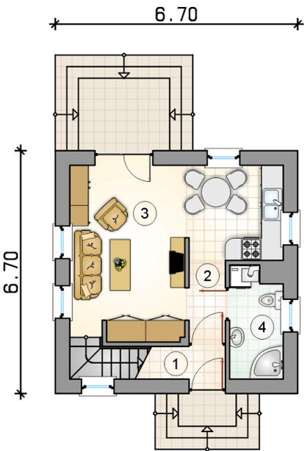
Rzut parteru
