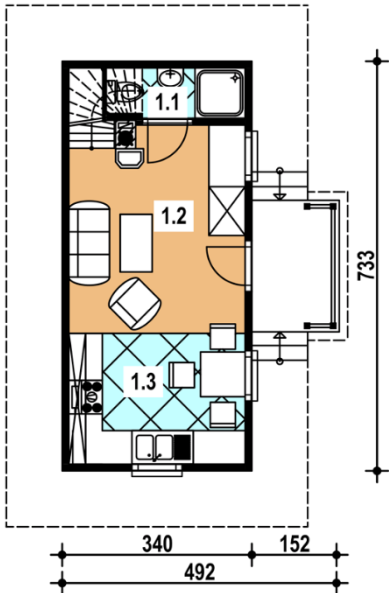
Rzut parteru
