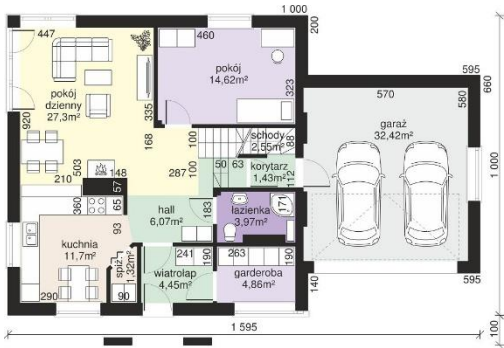
Rzut parteru
